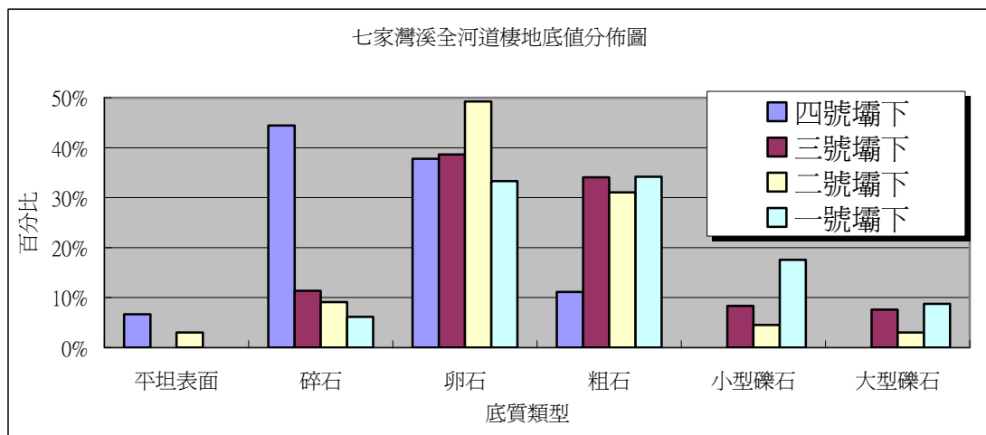
圖 3-62 七家灣溪河道棲地底質分佈圖
