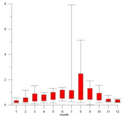
圖 3-17 七號壩之流量
