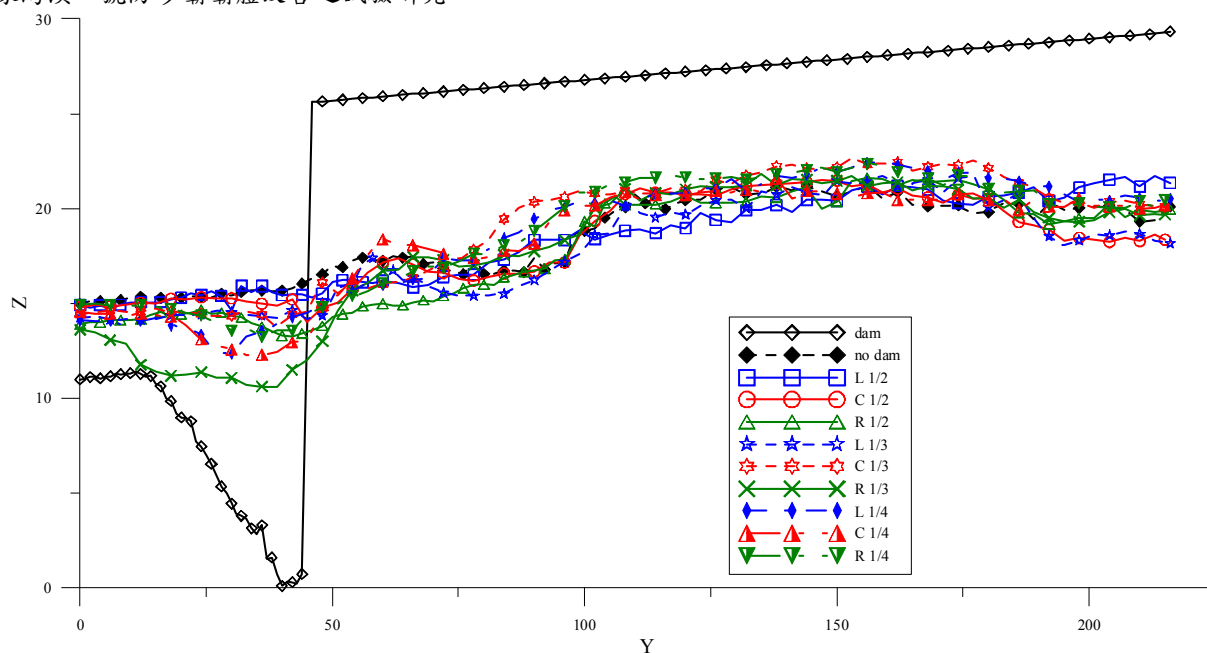
圖 3-42 防砂壩壩體不同改善方案改善前後之縱斷面變化(Q 50 )
