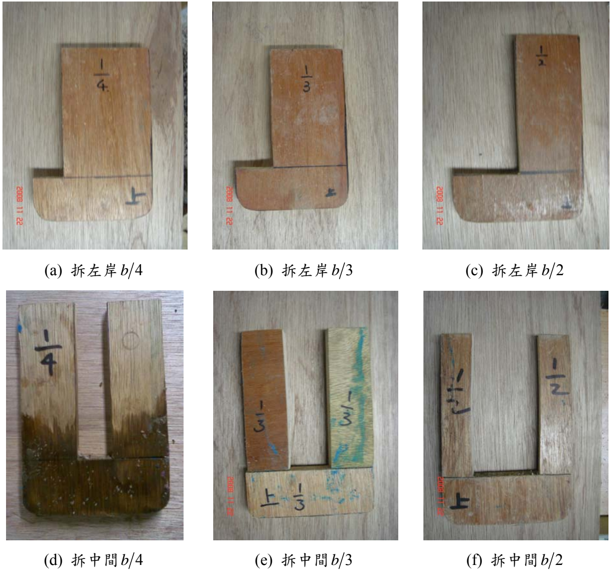
圖 3-32 壩體改善各方案之模型
