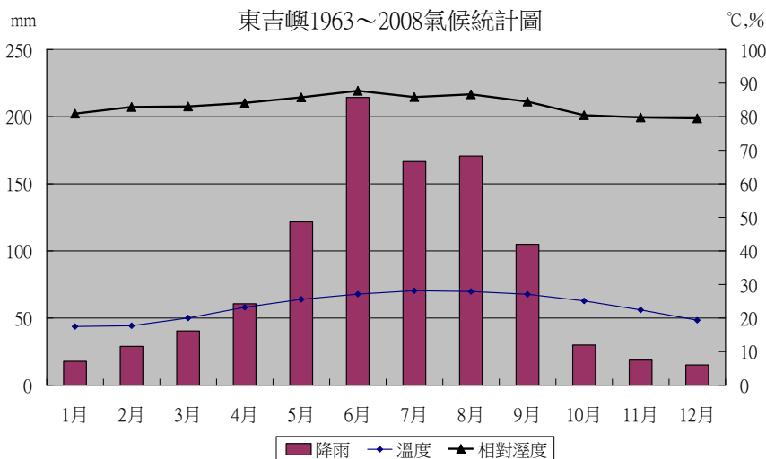
圖 2. 澎湖東吉嶼 1963~2008 氣候統計圖 (本研究整理，資料來源：中央氣象局)
