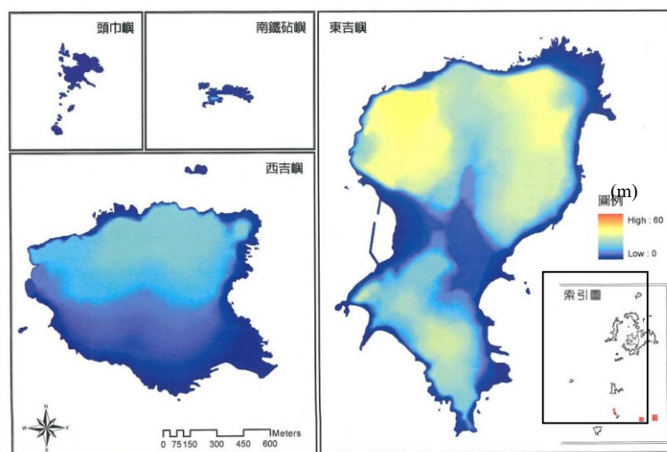
圖 3. 東吉嶼、西吉嶼、頭巾嶼及鐵砧嶼地形分析圖 (資料來源：中華民國永續發展學會 2008)
