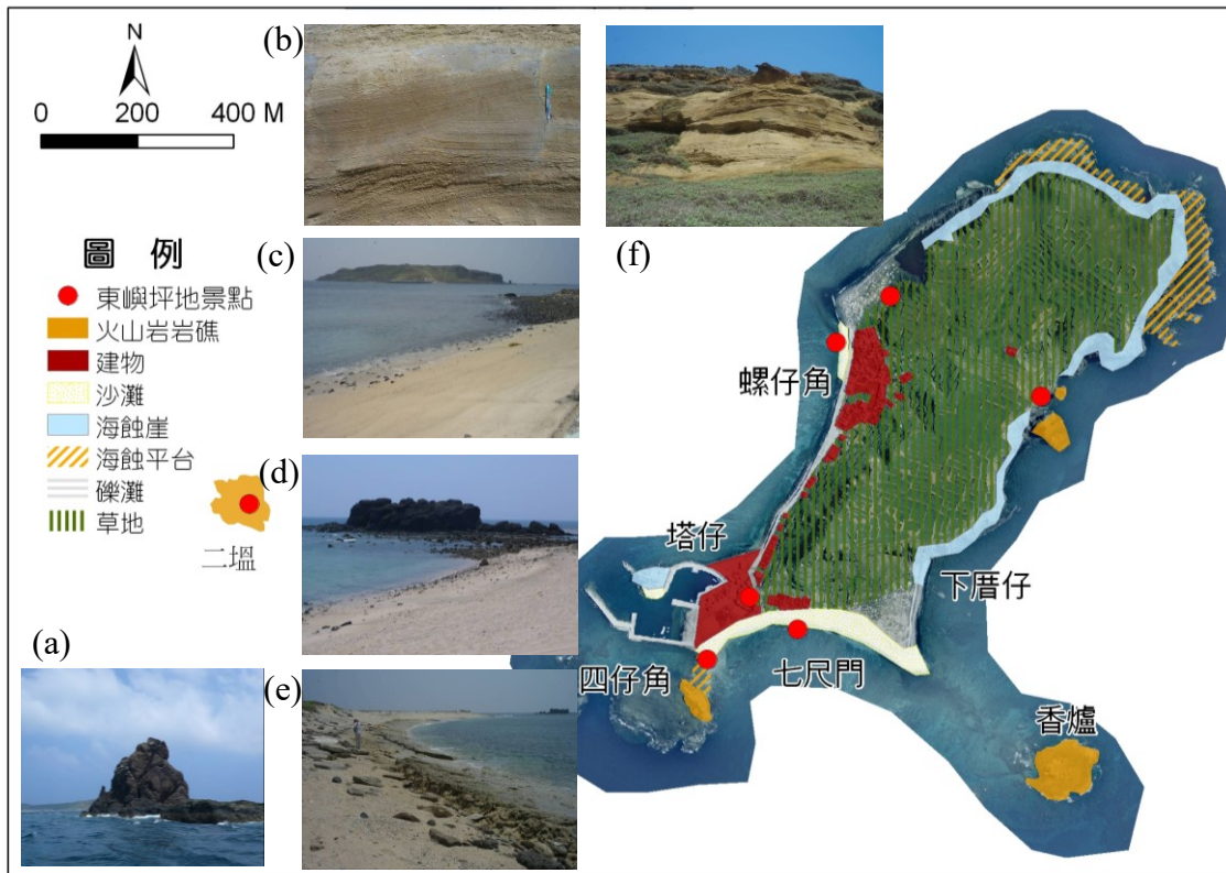
圖 7. 東嶼坪嶼、香爐及二塹景觀資源分佈圖
