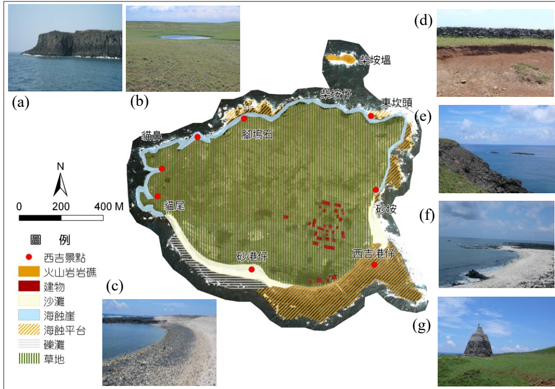
圖 5. 西吉嶼景觀資源分佈圖
