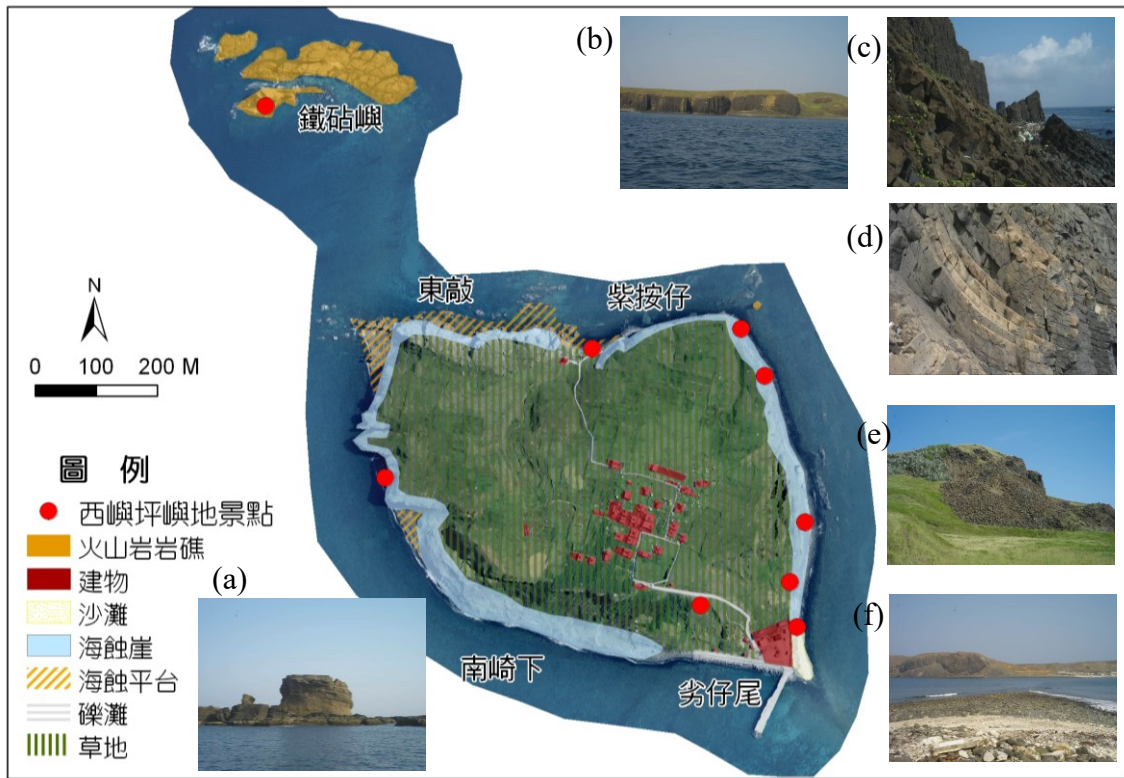
圖 6. 西嶼坪嶼及鐵砧嶼景觀資源分佈圖
