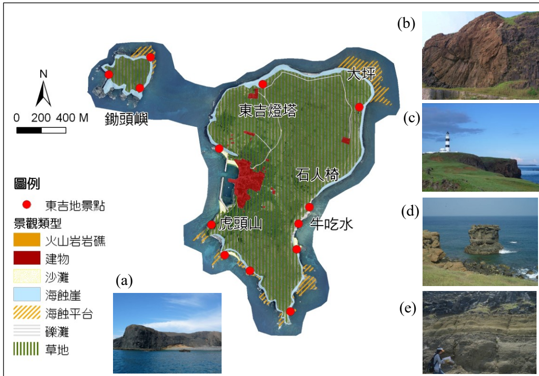
圖 4. 東吉嶼及鋤頭嶼景觀資源分佈圖
